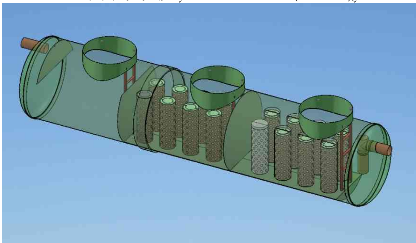
Рис. 1 Схема КСО «PromoТек-ОР-ОМ-SB» укомплектованного коалесцентными модулями ODG
