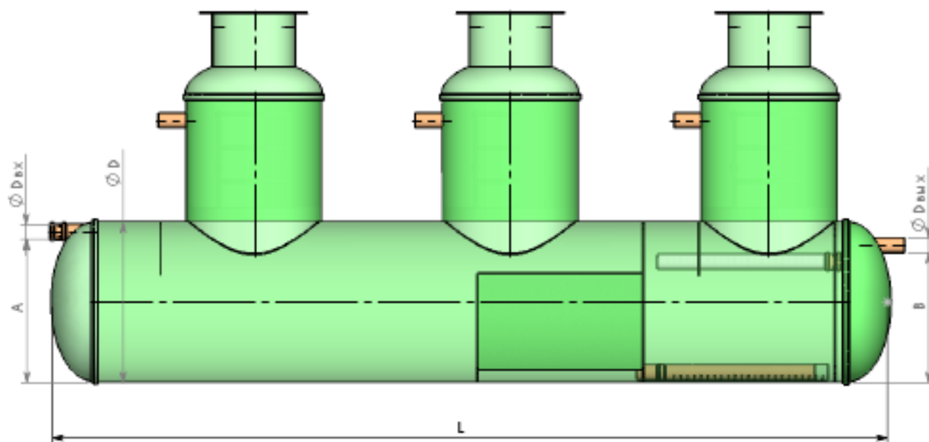
Рис. 1 Схема КСО «PromoТек-ОР-ОМ-SB» укомплектованного коалесцентными модулями ODG
