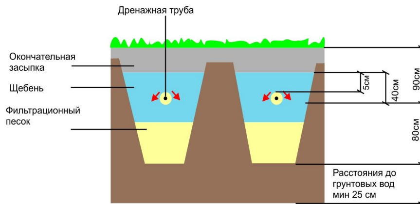
Рис. 4. Поперечное сечение поля фильтрации
