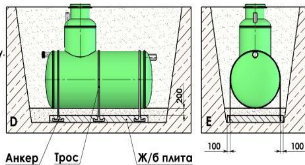
Установка в случае высокого уровня грунтовых вод
