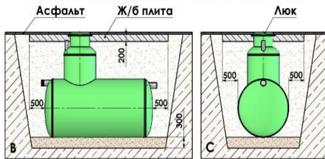
Установка в местах движения тяжелого транспорта
