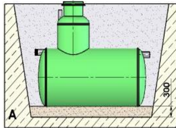
Установка вне пределов проезжей части
