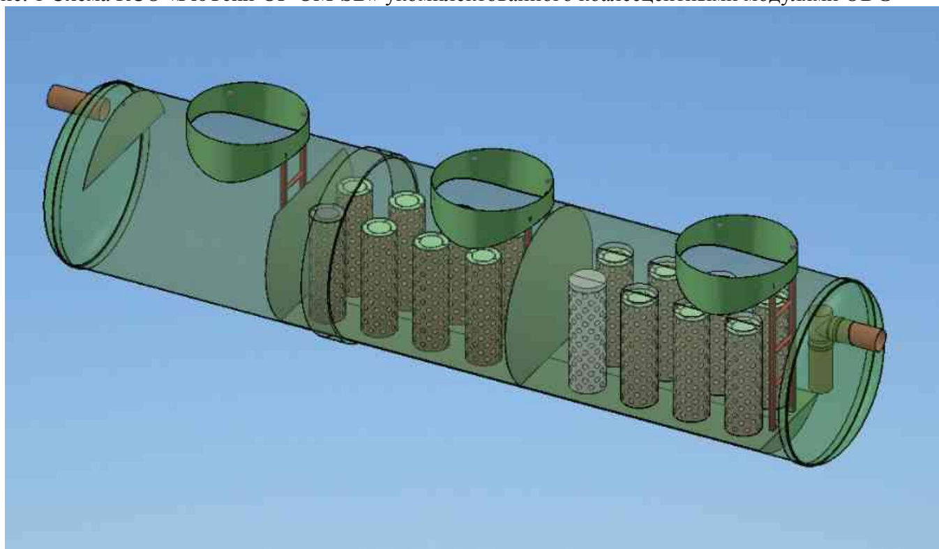
Рис. 1 Схема КСО «FloTenk-OP-OM-SB» укомплектованного коалесцентными модулями ODG
