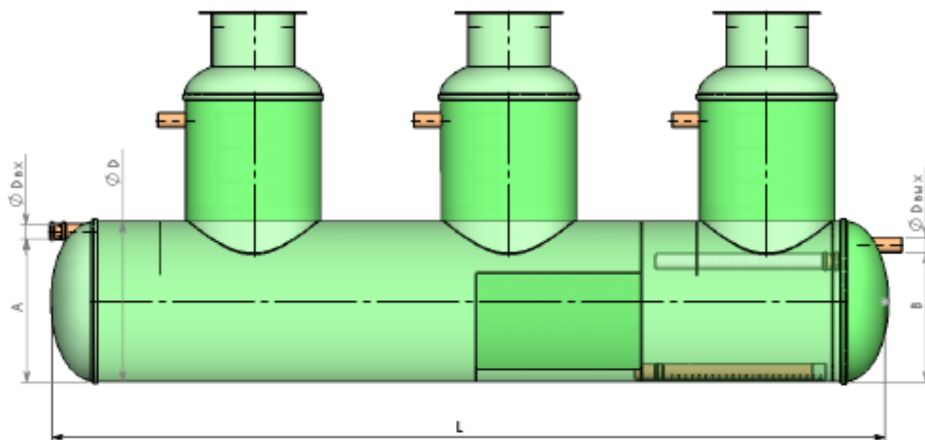
Рис. 1 Схема КСО «FloTenk-OP-OM-SB» укомплектованного коалесцентными модулями ODG
